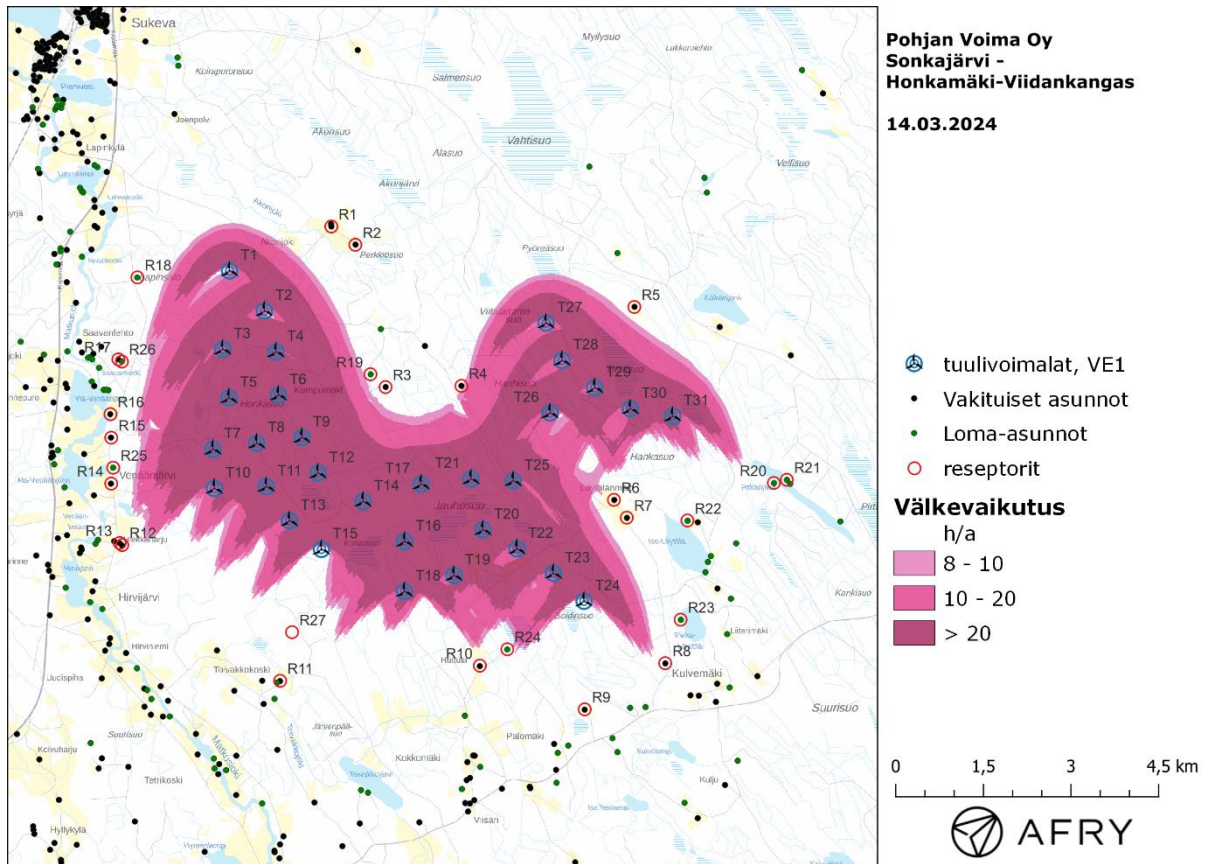
Kuva 3: Tuulivoimaloiden aiheuttama todennäköisen välkeen määrä ilman puuston vaikutusta.
