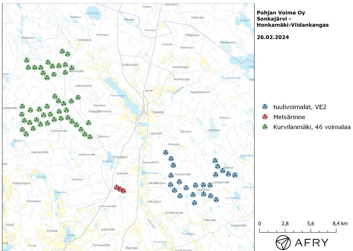
Kuva 4: Naapurivoimaloiden sijainnit suhteessa Honkamäki-Viidankankaan tuulivoimaloihin.
