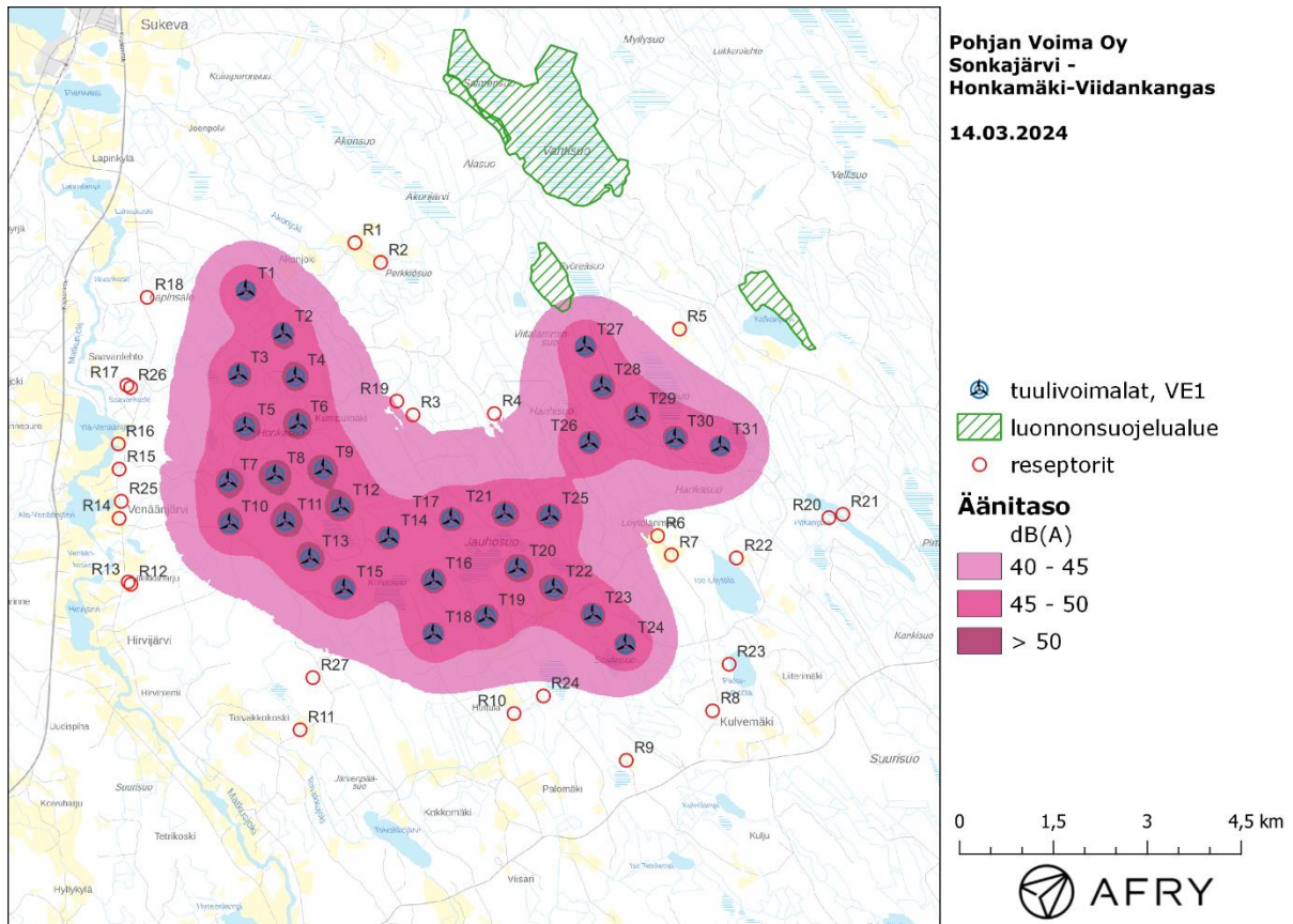
Kuva 4: Keskiäänitasot LAeq Honkamäki-Viidankankaan tuulivoimapuiston hankealueella.
