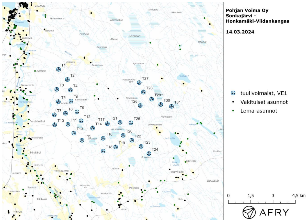
Kuva 1: Tuulivoimaloiden sijainnit Honkamäki-Viidankankaan hankealueella suunnitelmalla VE1.
