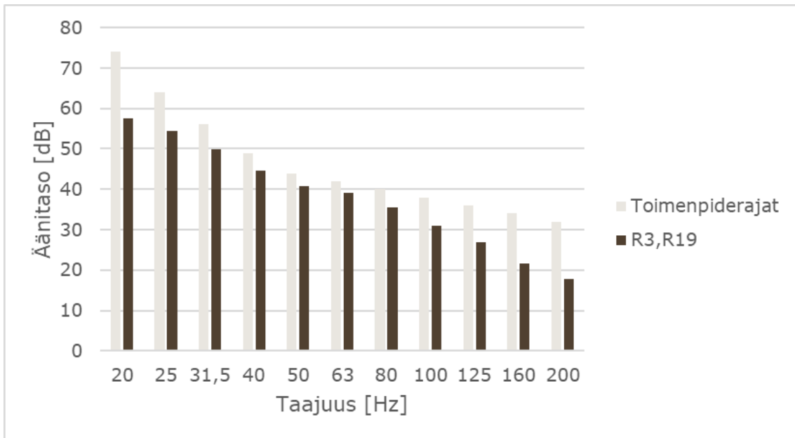
Kuva 5: Pienitaajuisten sisämelun tasot reseptorien R3 ja R19 kohdilla.
