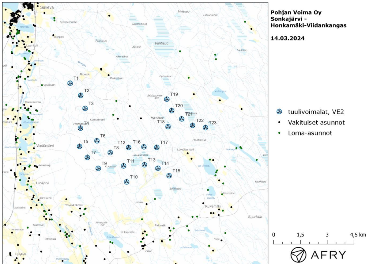
Kuva 1: Tuulivoimaloiden sijainnit Honkamäki-Viidankankaan hankealueella suunnitelmalla VE2.
