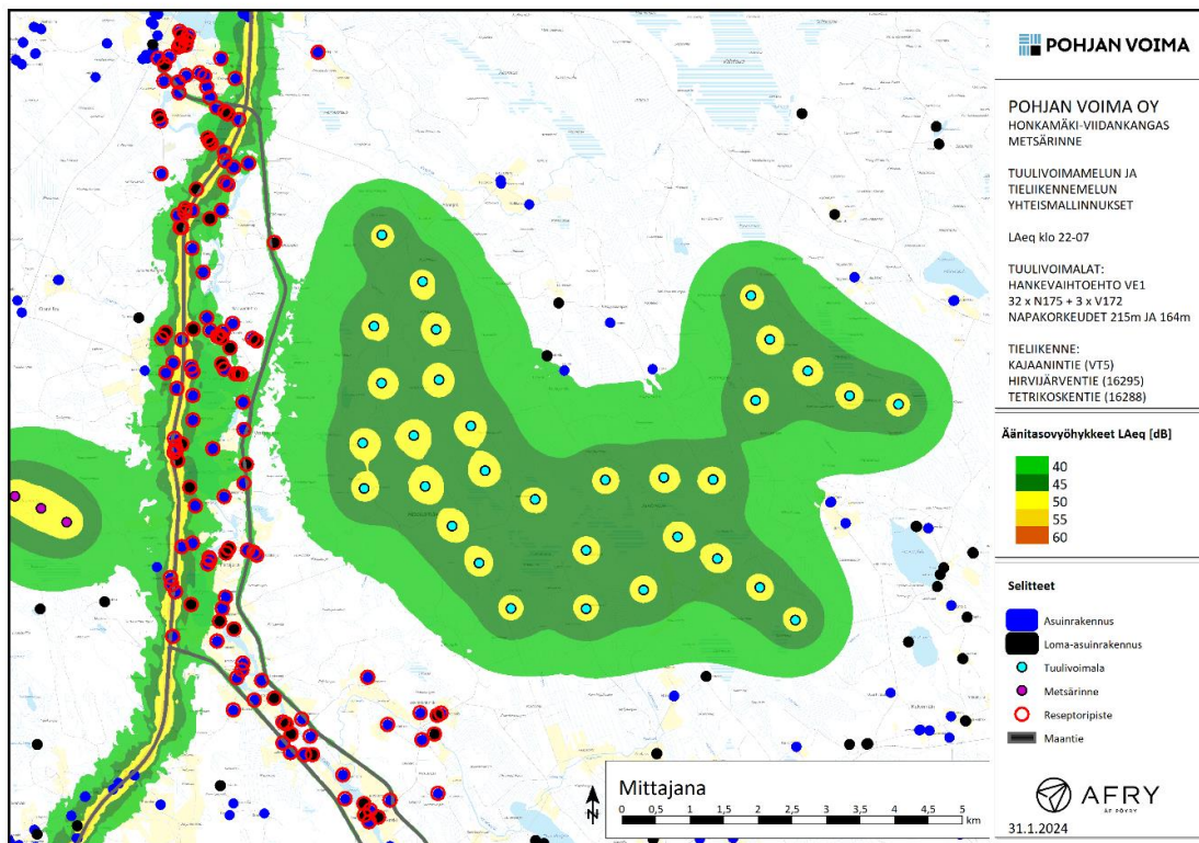
Kuva 10: Tuulivoimaloiden ja liikenteen aiheuttamat keskiäänitasot päiväaikaan (ylhällä) ja yöaikaan (alhaalla).
