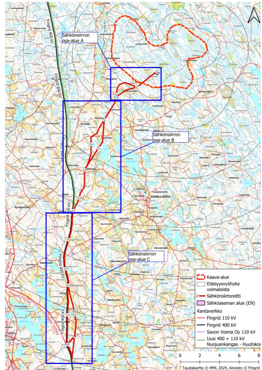
Kuva 4. Alustava suunnitelma sähkönsiirtovaihtoehdoista.
