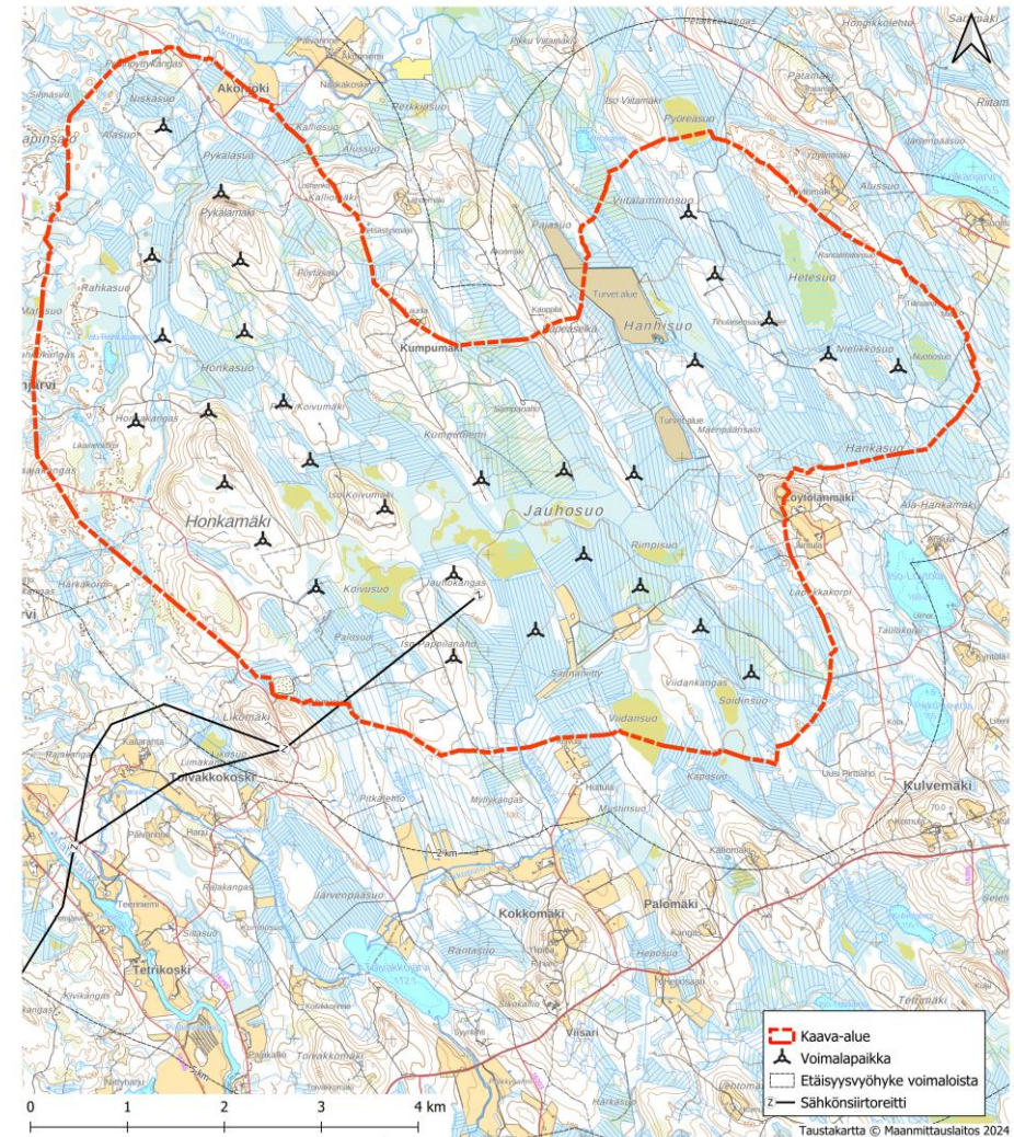
Kuva 3. Kaavaehdotuksen voimalapaikat kaava-alueella.
