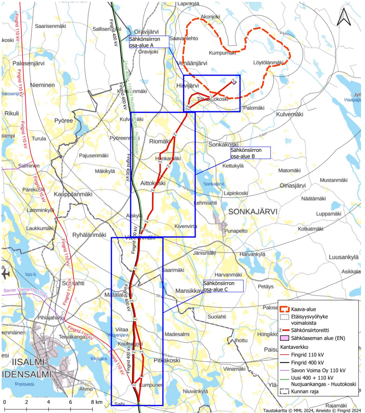
Kuva 25. Honkamäki-Viidankankaan tuulivoima-alueen suunniteltu sähkönsiirtoreitti.
