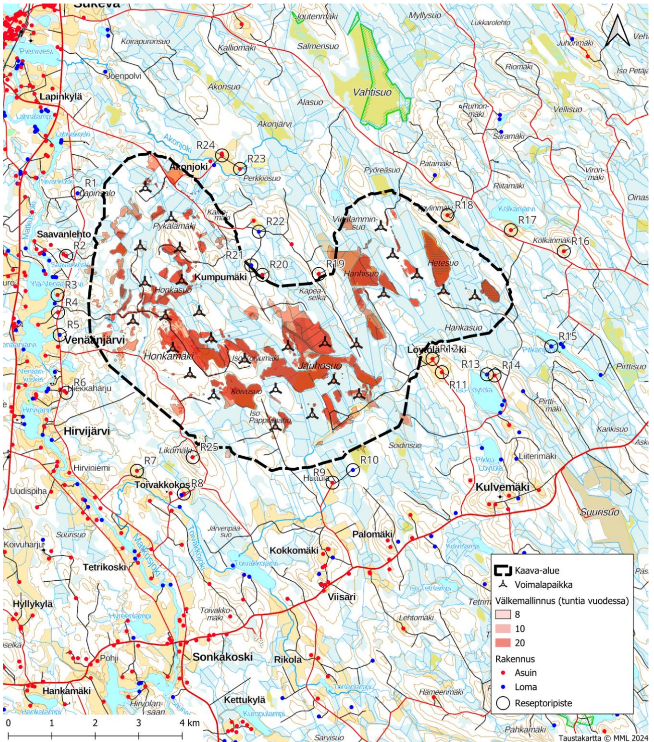
Kuva 32. Honkamäki-Viidankankaan tuulivoimaloiden aiheuttama todennäköisen välikkeen vuotuinen määrä, kun puuston välikettä vähentävä vaikutus huomioidaan mallinnuksessa.
