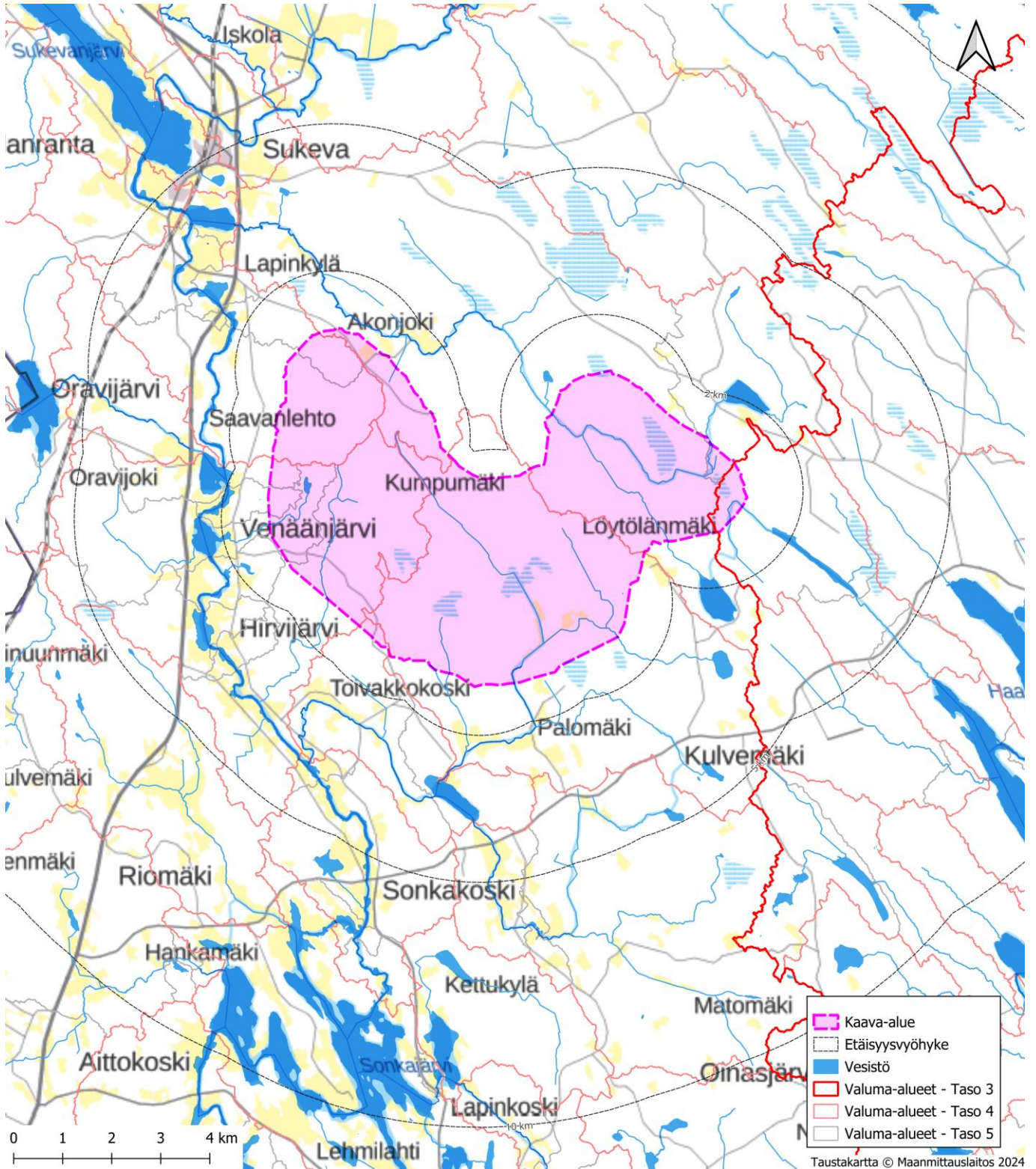
Kuva 14. Kaava-alueen ja lähiympäristön pintavedet ja valuma-alueet.
