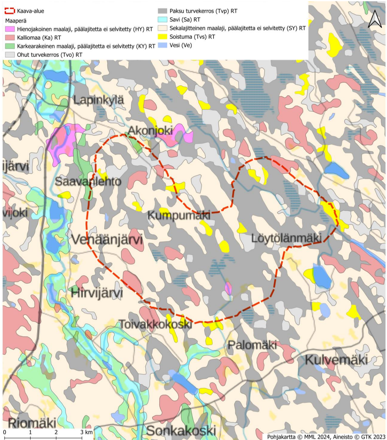
Kuva 15. Kaava-alueen maaperä (lähde: GTK).
