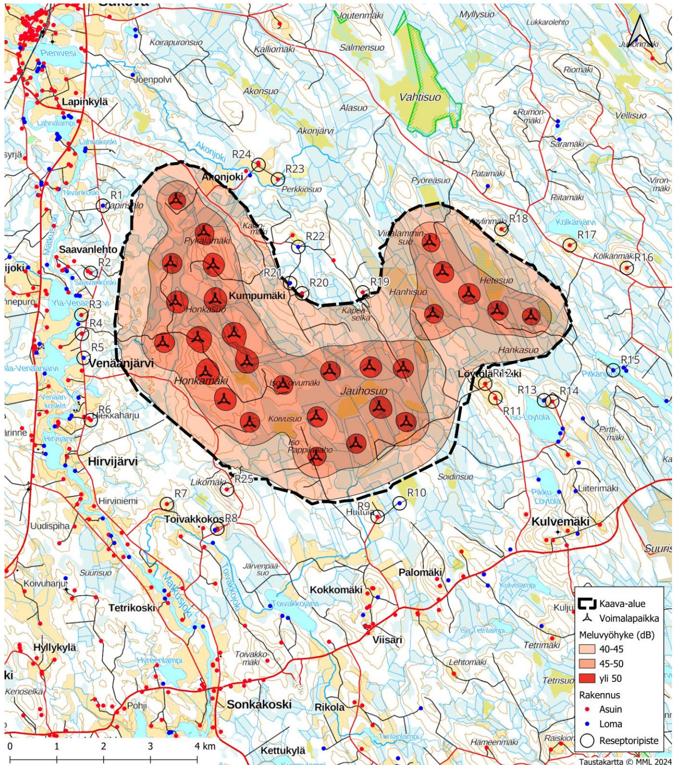
Kuva 32. Keskiäänitasot (LAeq) Honkamäki-Viidankankaan tuulivoimala-alueella kaavaehdotuksen voimalasijoittelulla.
