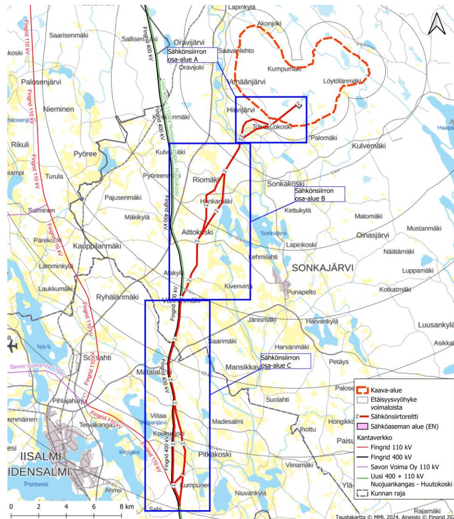
Kuva 4. Alustava suunnitelma sähkönsiirtovaihtoehdoista.
