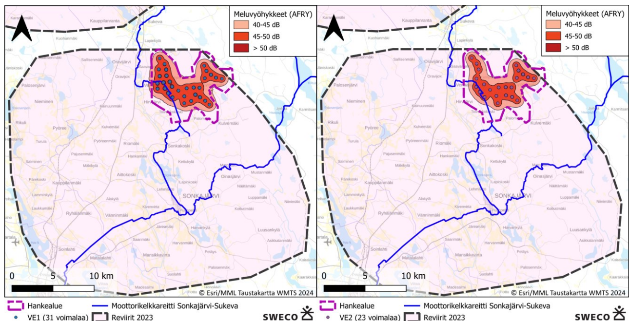
Kuva 29. Vasemmalla hankealueen melumallinnus hankevaihtoehdolla VE1 ja oikealla melumallinnus hankevaihtoehdolla VE2.
