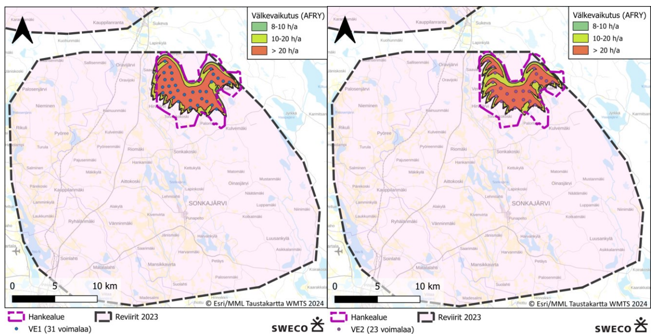
Kuva 30. Vasemmalla hankealueen välkemallinnus hankevaihtoehdolla VE1 ja oikealla välkemallinnus hankevaihtoehdolla VE2.
