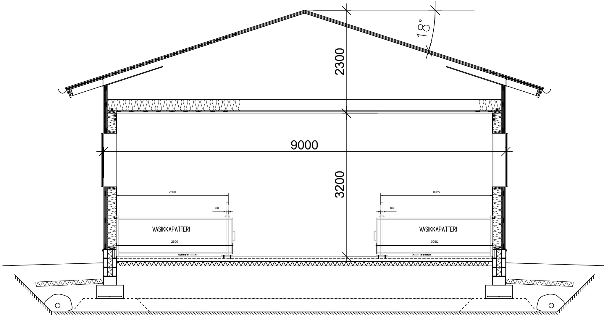
LEIKKAUS C-C
